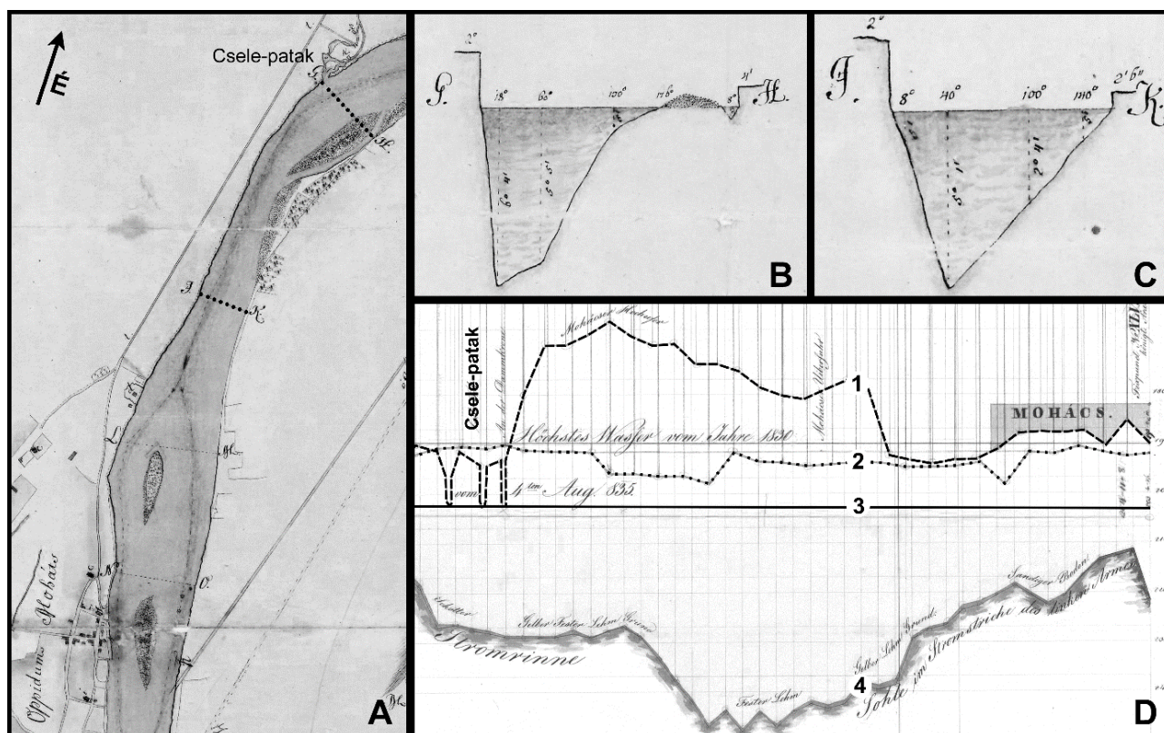
A Csele-patak torkolata alatti Duna-szakasz, valamint a meder keresztmetszetei (1808) és a partélek hosszmetzete (1830–1840) (Magyar Nemzeti Levéltár Országos Levéltára, L S 12 div. XIII. No. 370; Uo. OL S 80 Duna No. 57/1-29.)
